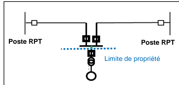
SCHEMA 3 : Raccordement par une liaison et un poste en coupure sur une liaison existante
